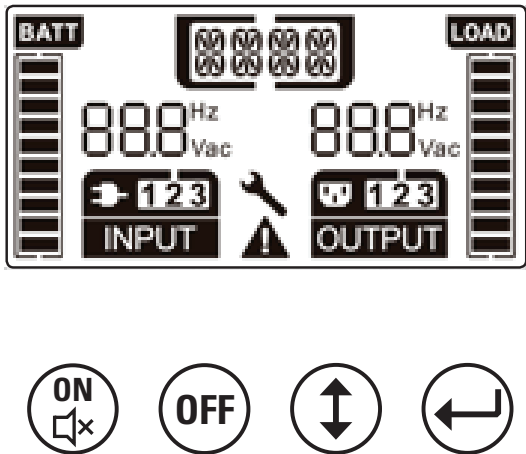
Abb. 13. Bedienfeldansicht.
