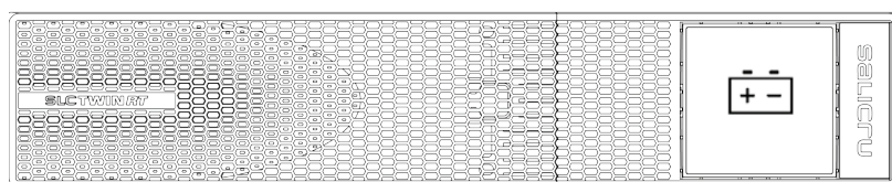
Abb. 1. Frontansichten der Modelle von 0,7 bis 10 kVA und ihre Batteriemodule für erweiterte Autonomie.
