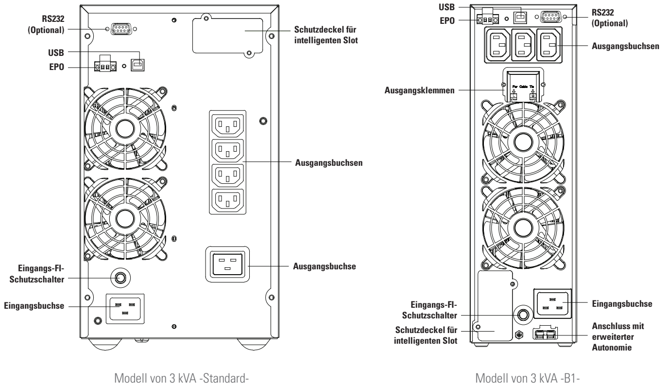
Abb. 5. Rückansichten, Modell von 3 kVA mit IEC-Ausgangssteckern.
