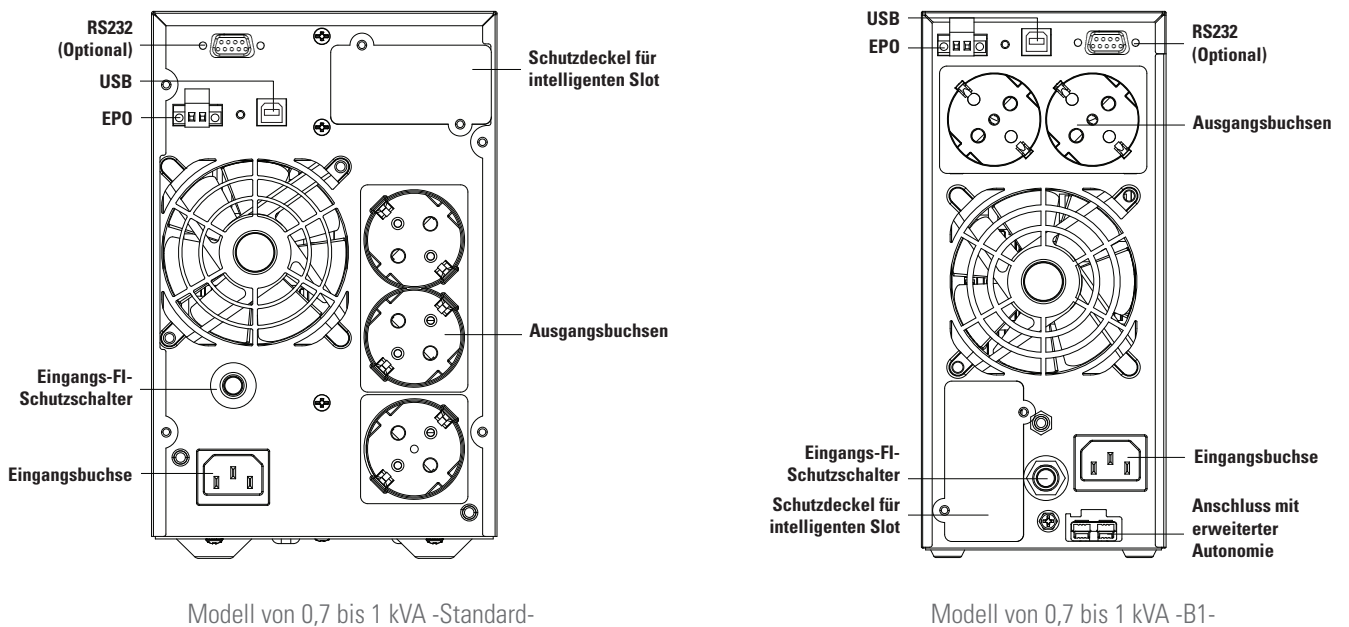
Abb. 6. Rückansichten, Modelle von 0,7 bis 1 kVA mit Schuko-Ausgangsbuchsen.
