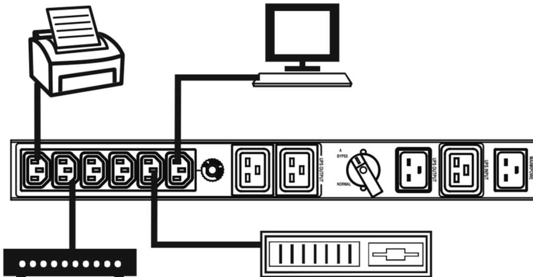
Abb. 5: Steckdose am PDU-Bypass für periphere Geräte wie Bildschirm, Drucker oder Switches (Slave)
