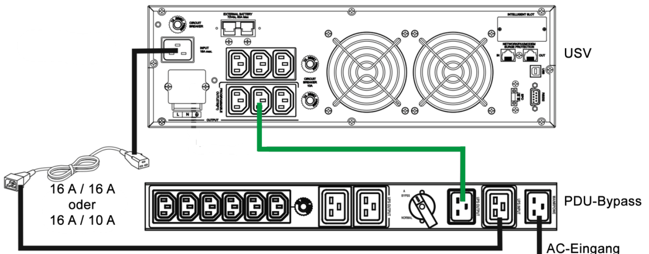
Abb. 4: Anschlüsse zwischen PDU-Bypass und USV. Schwarzer Strich USV-Eingang und grüner Strich USV-Ausgang.
