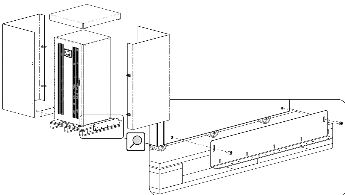
Abb. 2: Vorgehen beim Abheben der USV von Palette
