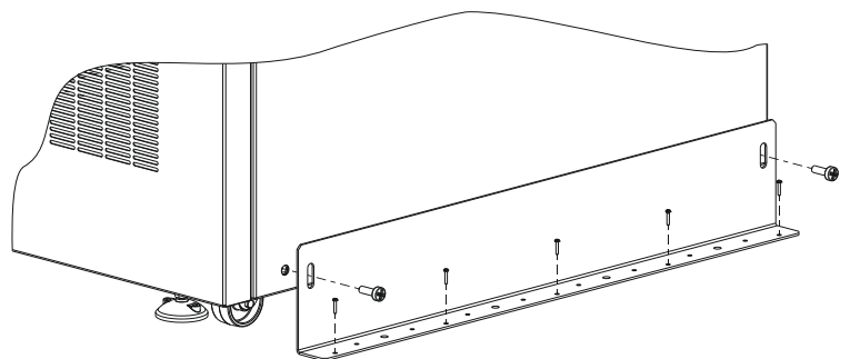
Abb. 4: Halterungen für Befestigung
