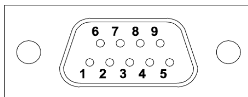
Abb. 12: RS232-Stecker
