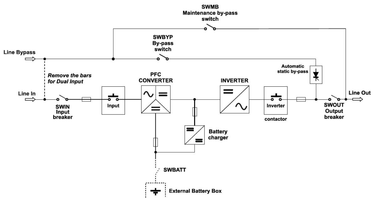
Abb. 10: Blockscheema der USV
