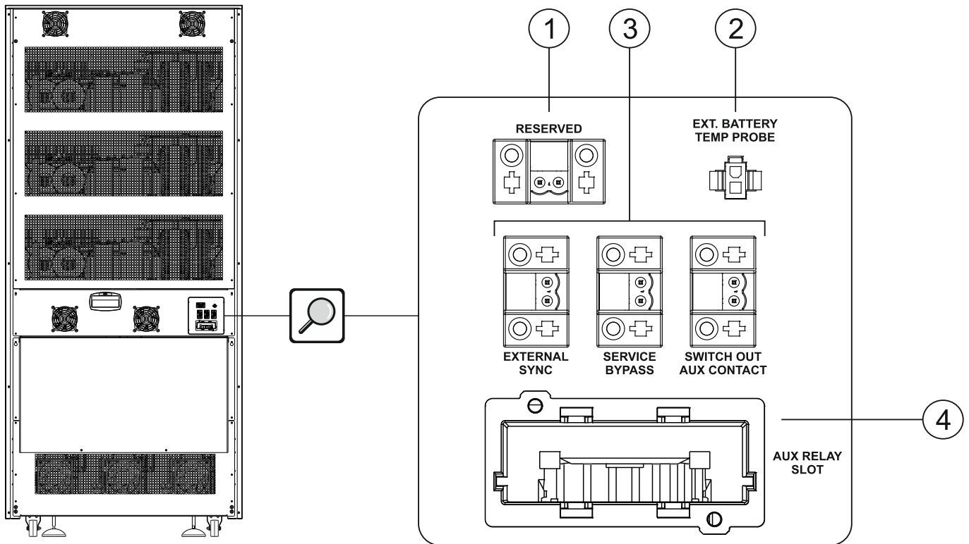
Abb. 14: Details mit den Kommunikationsschnittstellen.
