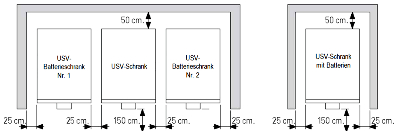
Abb. 5: Abmessungen der USV
