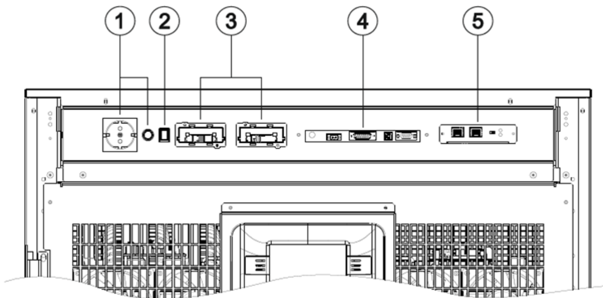
Abb. 6: Benutzeroberfläche (Vorderseite)
