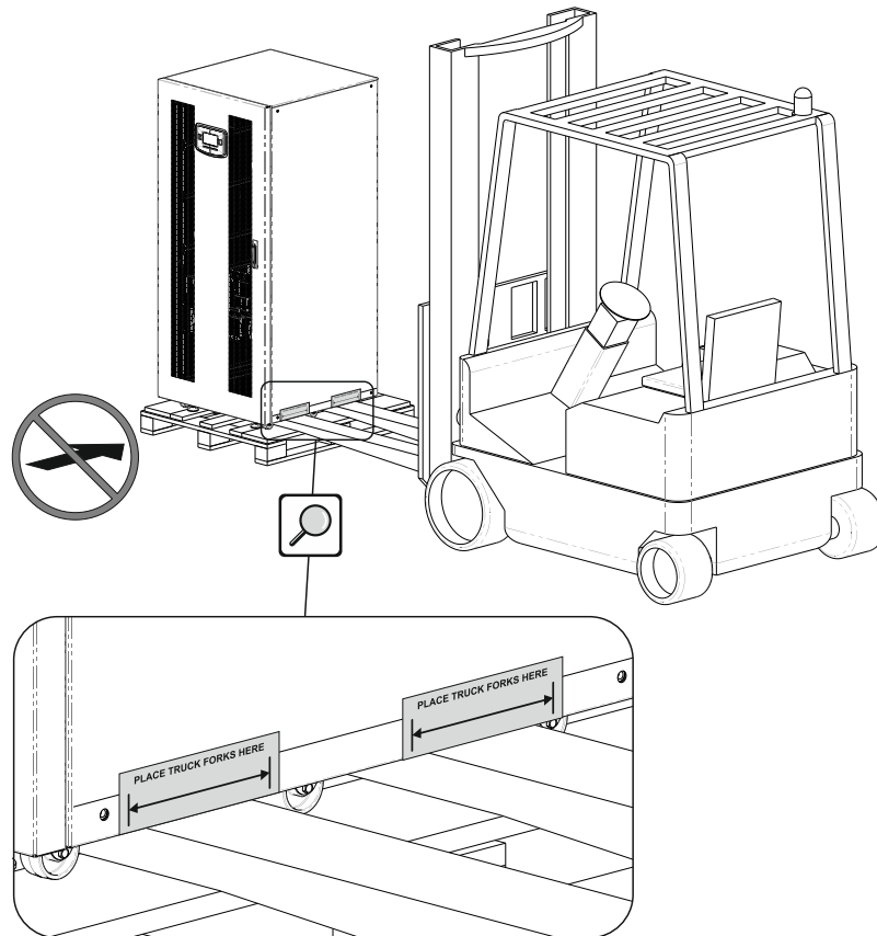
Abb. 3: Groupys GM von Palette heben
