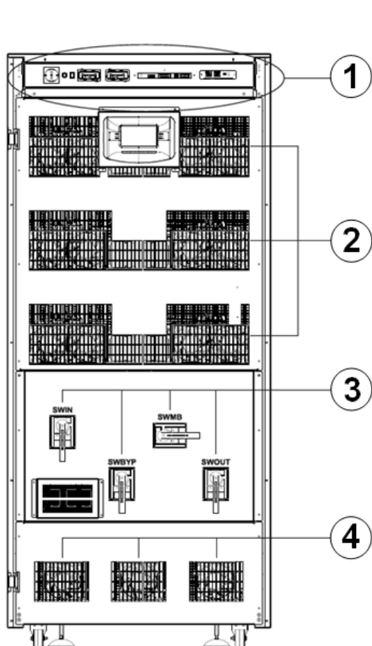
Abb. 7: Vorderansicht
